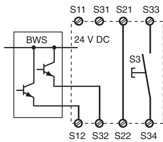
Fig. 8: Lichtschrankensteuerung, zwei-kanalig, Querschlußerkennung durch BWS, überwachter Start/Dual-channel light curtain control, short circuit detection via ESPE, monitored reset/Comande par 2 canaux par barrage immatériel, surveillance du poussoir de validation
