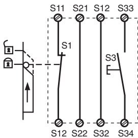
Fig. 5: Control de puerta de protección monocal, rearme supervisado/Comando riparo mobile monocale, start controllato/Eenkanalige hekbewaking, bewaakte start
