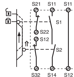
Fig. 7: Control de puerta de protección bicanal, rearme automático/Comando riparo mobile bicanale, start automatico/Tweekanalige hekbewaking, automatische start
