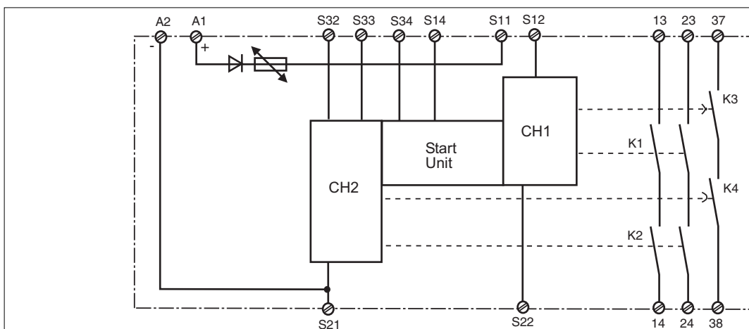
Fig. 1: Esquema de conexionado interno/Schema di collegamento interno/Intern schema
