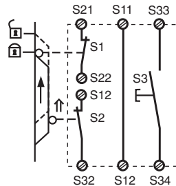
Fig. 6: Control de puerta de protección bicanal, rearme supervisado/Comando riparo mobile bicanale, start controllato/Tweekanalige hekbewaking, bewaakte start
